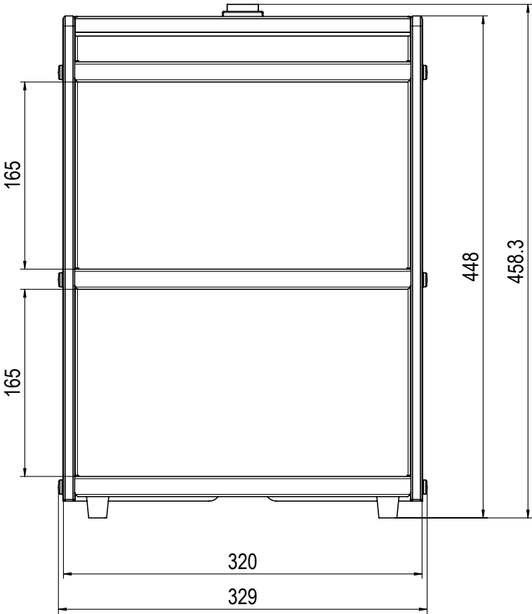
Vooraanzicht
