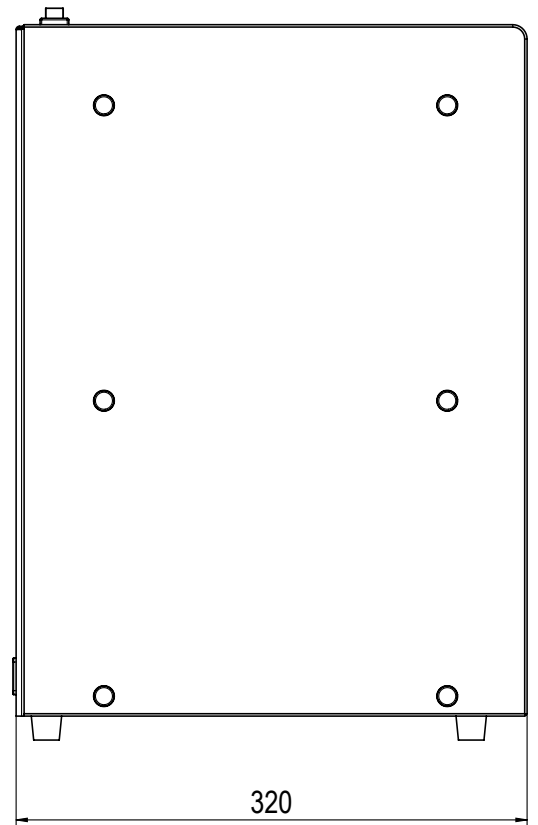
Från sidan
