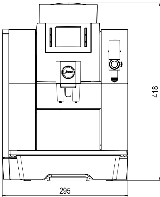
Vista verticale
