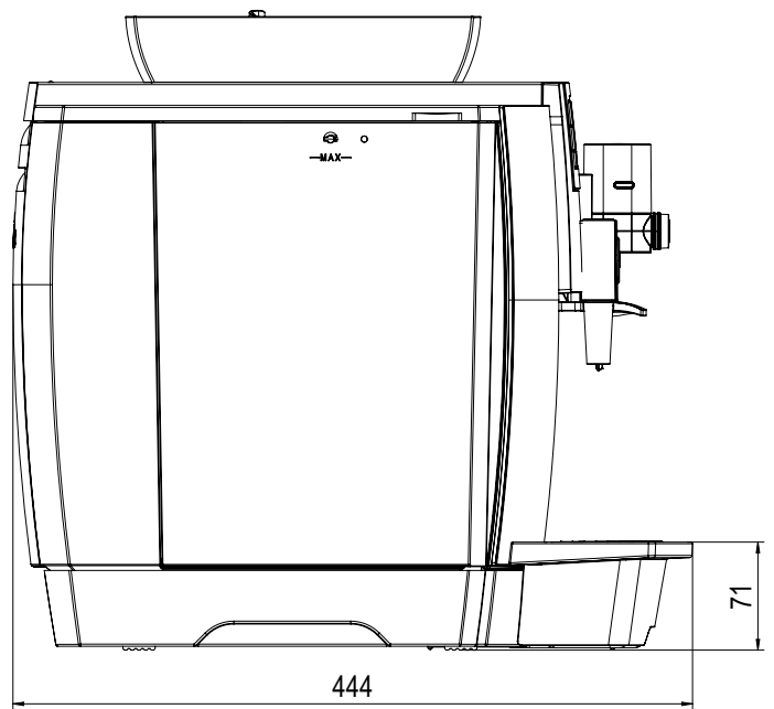
Vista laterale
